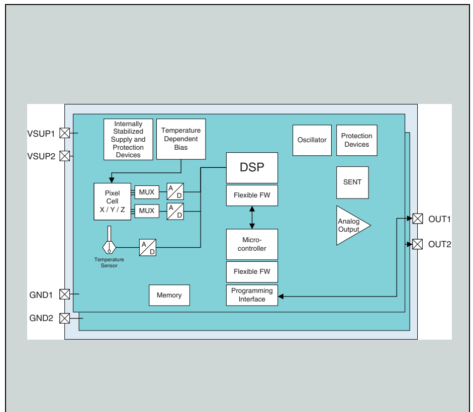
Fig. 1: Block diagram of the HAR 3927
